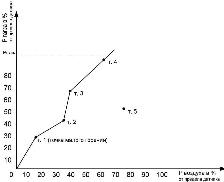
Рис. 3. График соотношения газ-воздух.
