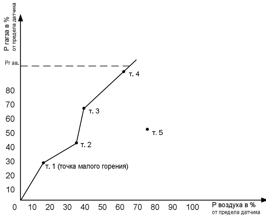
Рис. 3. График соотношения топливо-воздух.
