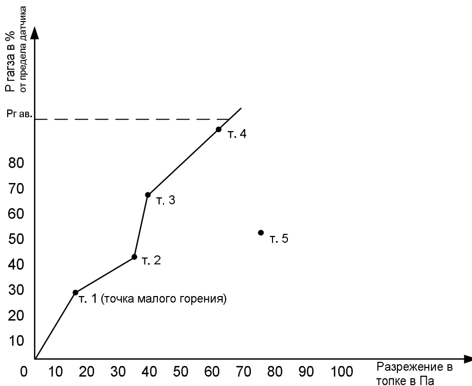
Рис. 3. График соотношения газ-разрежение.
